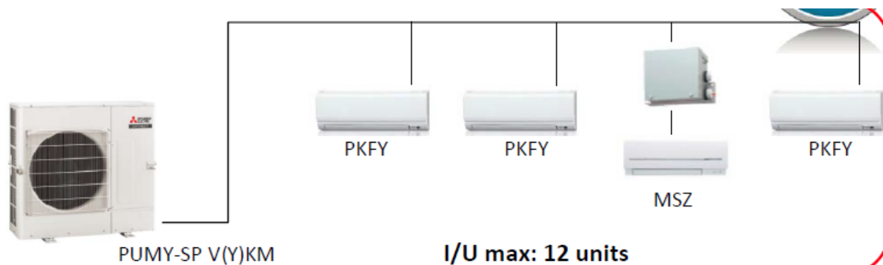
Skenari 1:Njesi VRF +LEVkit
