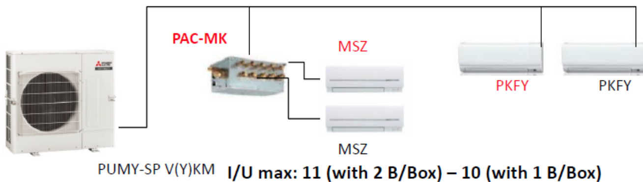
Skenari 3:Njesi VRF + Njesi multi me branch box
